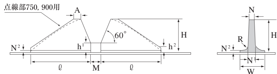
クライマー寸法表(I)
