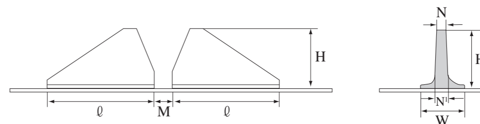
クライマー寸法表(III)
