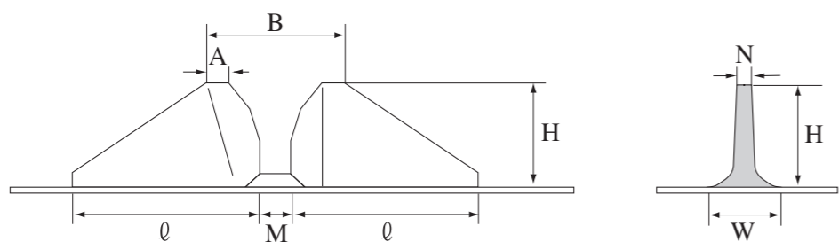
クライマー寸法表(II)
